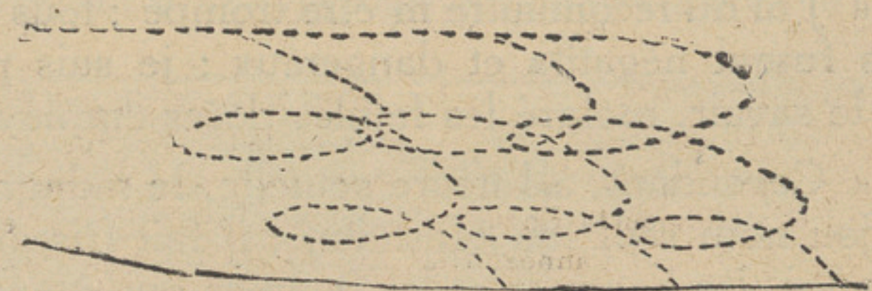
Ce schéma montre le mouvement hélicoïdal et oscillatoire des éléments détritiques au cours de leur propagation vers le fond de la mer.
