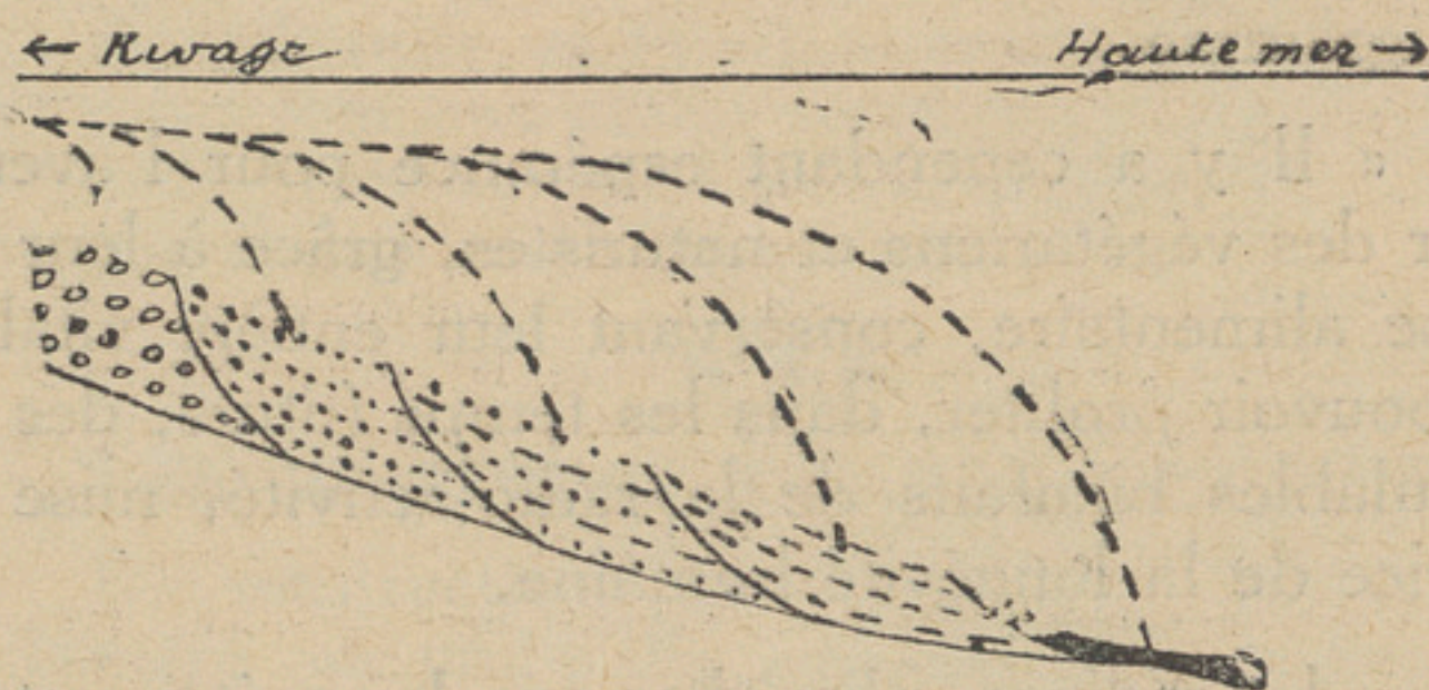
Ce schéma montre, de gauche à droite, les cailloux, les sables, les sables argileux, les boues argileuses et organiques se déposant de plus en plus loin du rivage.
